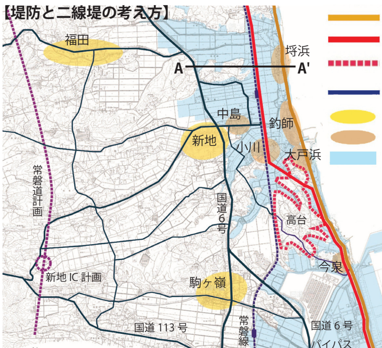
【A-A'断面】 10m以上の区域で安全な場所で丘陵状堤防、公園、防潮堤 国道6号 住宅再建 JR常磐線再建 二線堤の整備 防潮林等
